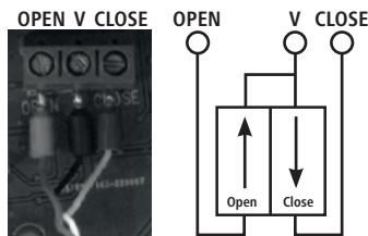
Tilslutningsklemmer til eksterne trykknapper
