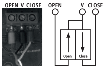
Anslutningsklämmor för extern knapp
