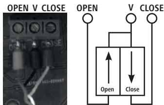
Ulkaisen näppäimen liittinisko
